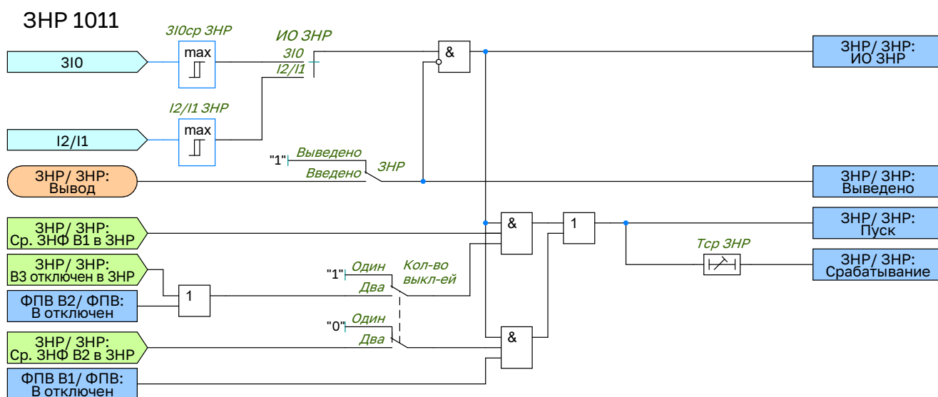
Рисунок 2.57 – Функциональная схема логики ЗНР
