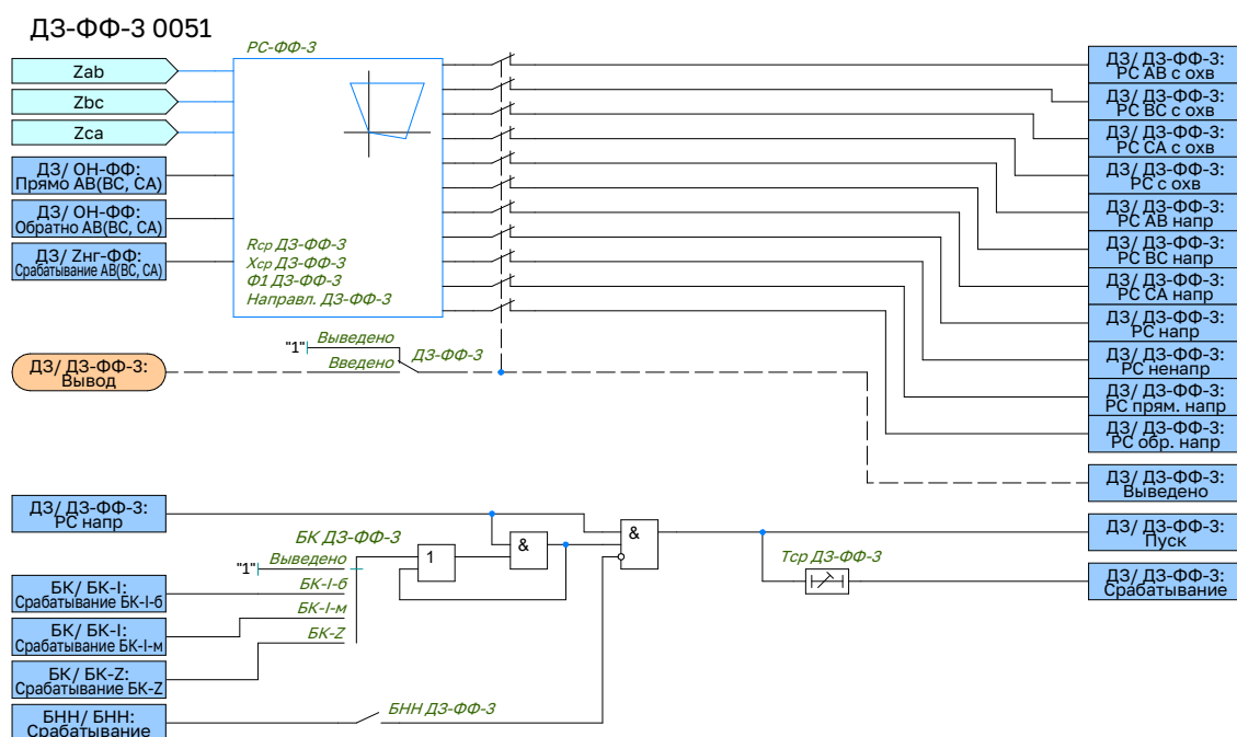
Рисунок 2.34 – Функциональная схема логики ДЗ-ΦФ-3
