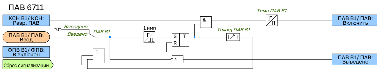
Рисунок 2.72 – Функциональная схема логики ПАВ
